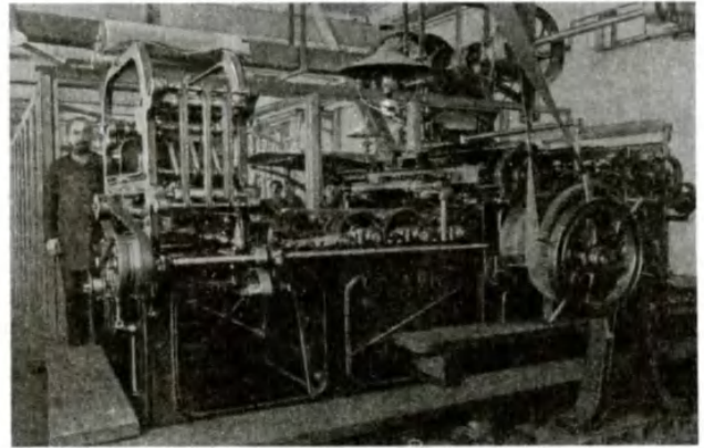
Ротационная печатная машина в типографии Товарищества печатного дела и торговли И. Н. Кушнерёв и К о .
